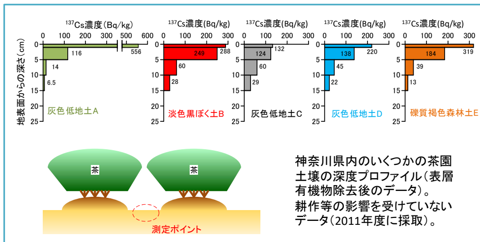
図 13 神奈川県の茶畑における放射性セシウムプロファイル
