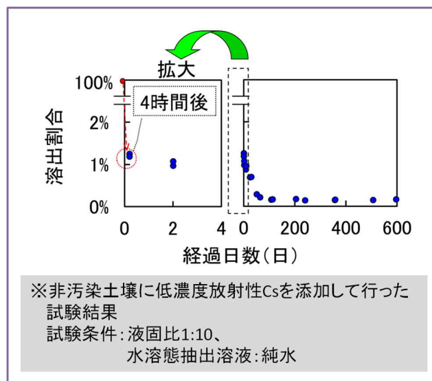
図6 土壌中（黒ボク土）の放射性セシウム（水溶性）の割合の経時変化
